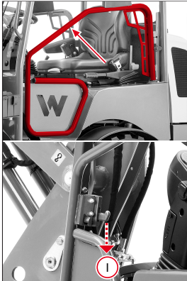
Abb. 42: Rückhaltesystem öffnen und schließen
