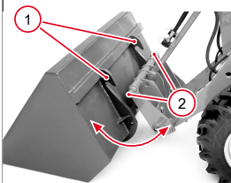
Abb. 105: Anbaugerät an- kuppeln
