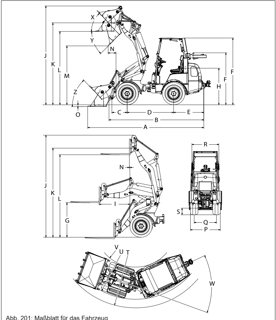
Abb. 201: Maßblatt für das Fahrzeug
