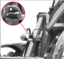
Abb. 125: Steckdose an der Ladeanlage
