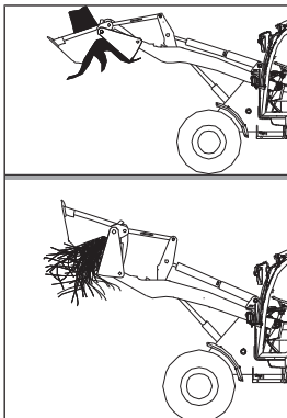
Abb. 136: Große, sperrige Gegenstände greifen
