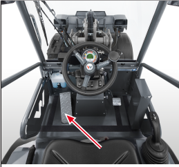
Abb. 72: Fahrzeug bremsen
