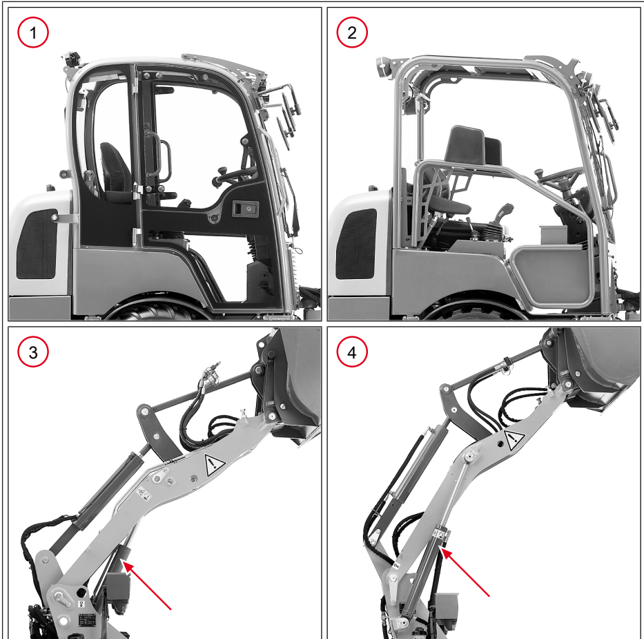
Abb. 207: Ausstattungsvarianten
