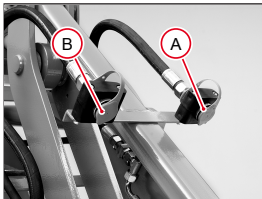
Abb. 113: Standard-Hydraulikanschlüsse bedienen
