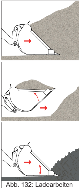
Abb. 132: Ladearbeiten
