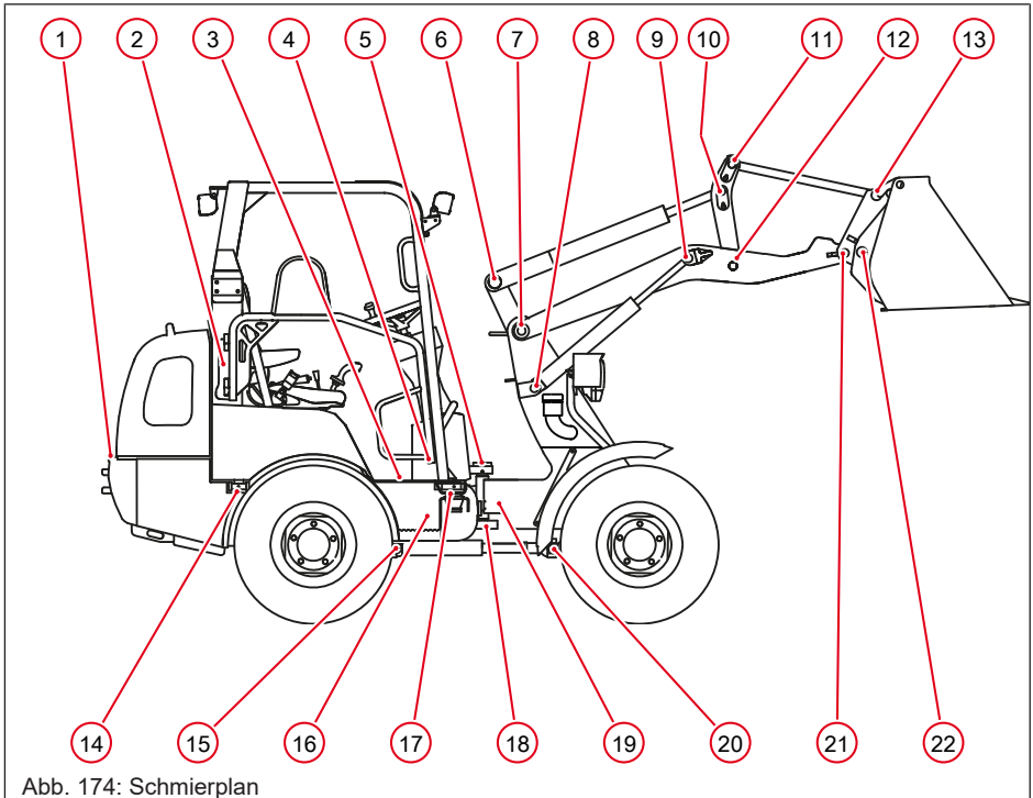
Abb. 174: Schmierplan
