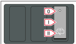
Abb. 86: Schalter für Scheibenwischer hinten
