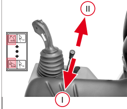
Abb. 113: Standard-Hydraulikanschlüsse bedienen
