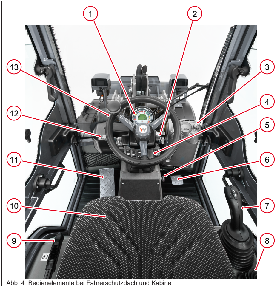
Abb. 4: Bedienelemente bei Fahrerschutzdach und Kabine
