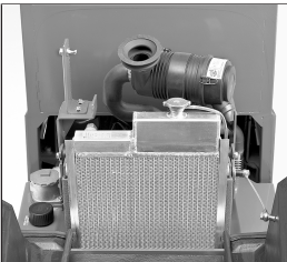
Abb. 182: Kühler im Motorraum
