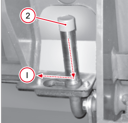
Abb. 104: Anbaugerät an- kuppeln mit mechani- scher Verriegelung
