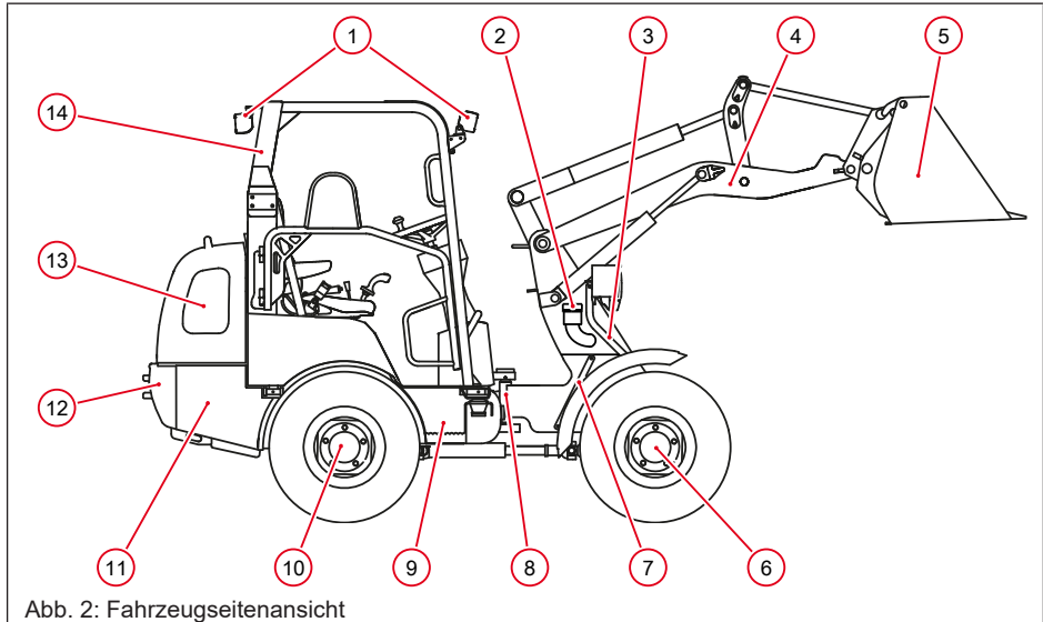
Abb. 2: Fahrzeugseitenansicht
