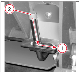
Abb. 106: Mechanische Verriegelung verriegeln
