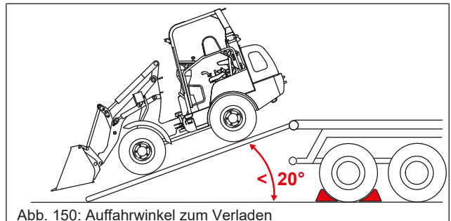
Abb. 150: Auffahrwinkel zum Verladen
