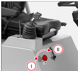
Abb. 71: Handinrichtung bedienen
