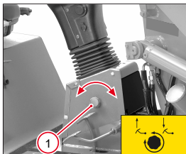
Abb. 62: Leerlaufdrehzahlverstellung
