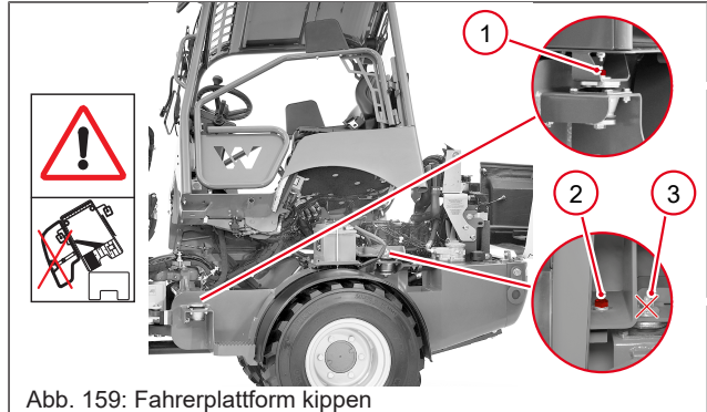
Abb. 159: Fahrerplattform kippen
