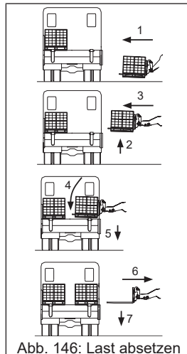
Abb. 146: Last absetzen
