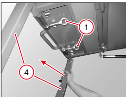
Abb. 97: Fahrerschutzdach in Schutzstellung bringen
