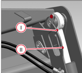
Abb. 135: Orientierungshilfen an der 4-in-1-Schaufel
